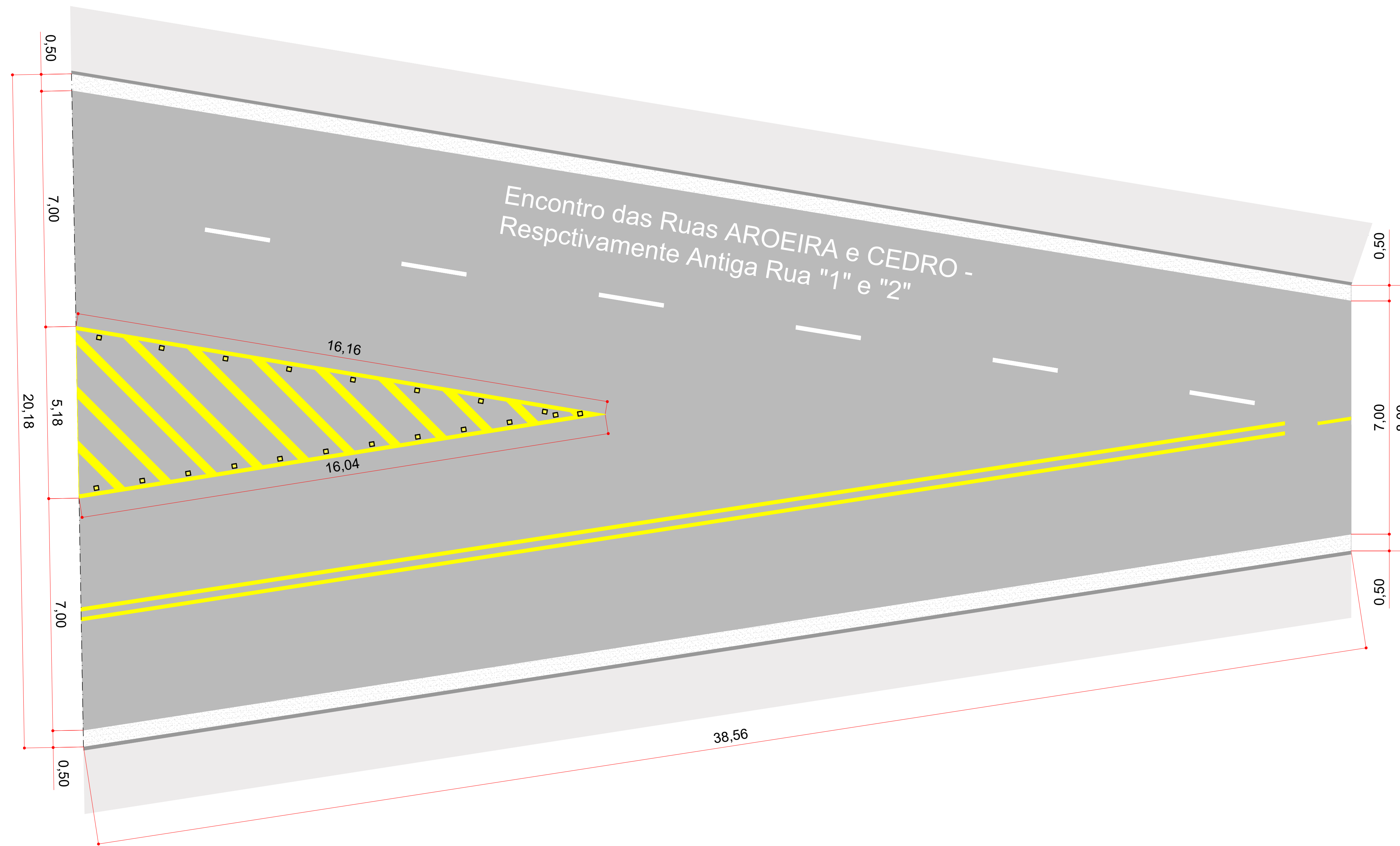
Detalhamento do encontro das vias ENCONTRO DAS RUAS AROEIRA E CEDRO Escala 1:75 Cotas: m
