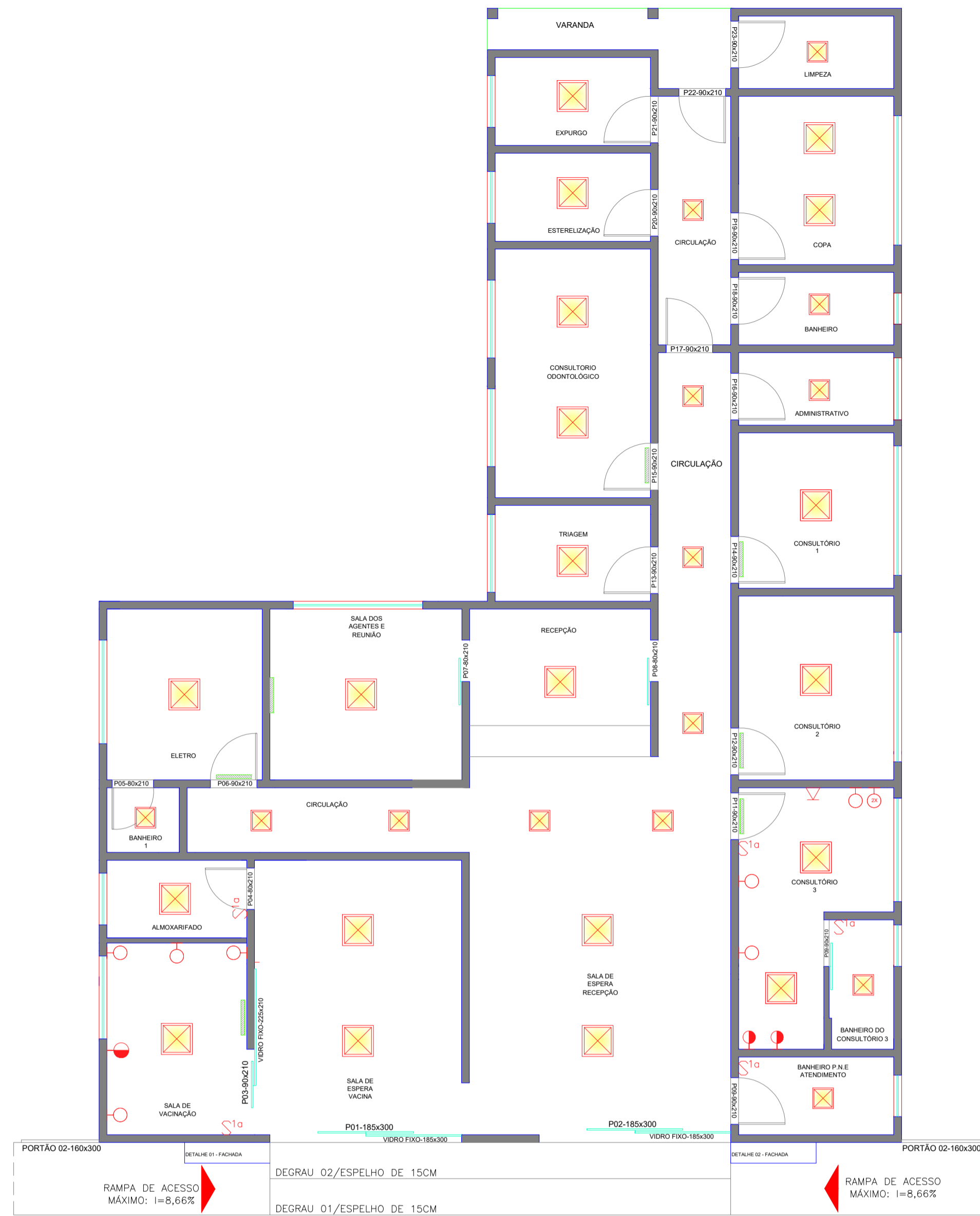
PONTOS DE ÁGUA FRIA E BANCADAS ESC. 1:50
