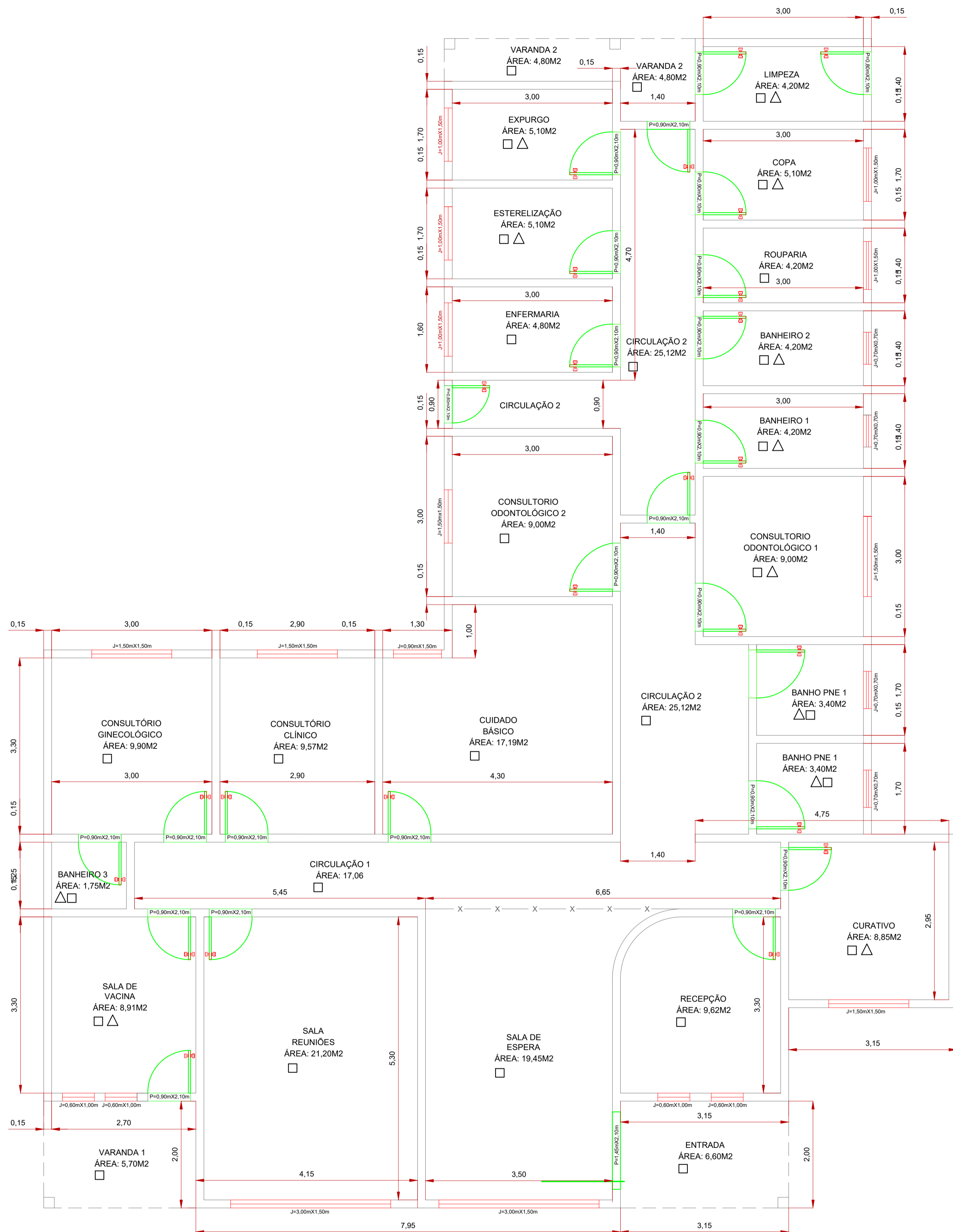
PLANTA BAIXA DE DEMOLIÇÕES E RETIRADAS ESC. 1:50
