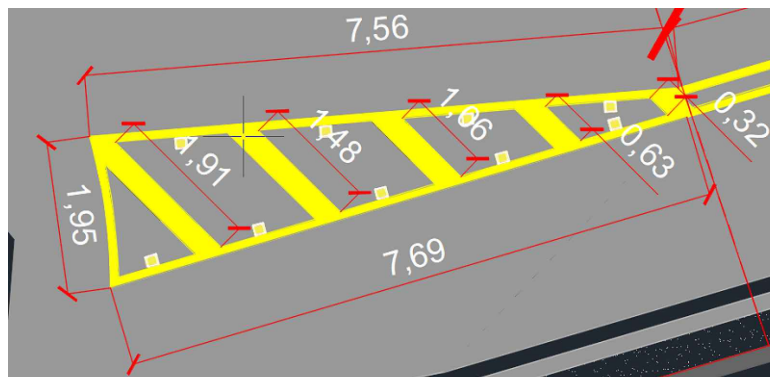
Detalhamento da zebra de preenchimento da área de pavimento não utilizável Cotas: m Linhas de 0,30m = 5,40m x 0,30m = 1,62m² Linhas de 0,10m = 17,20m Tachas refletivas: 9 unidades
