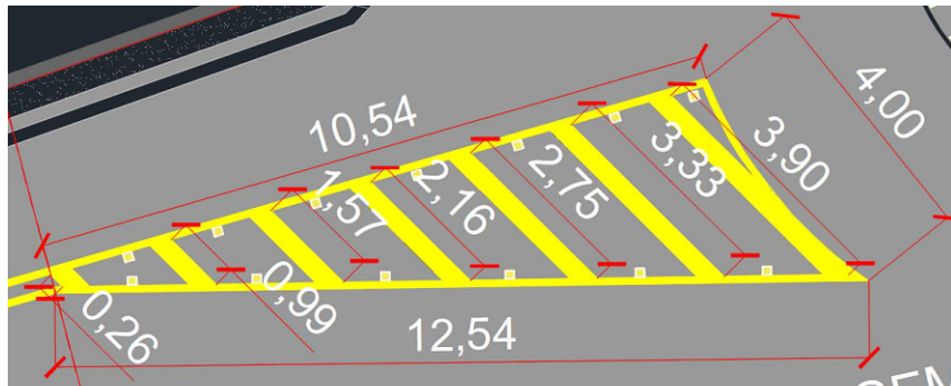
Detalhamento da zebra de preenchimento da área de pavimento não utilizável Cotas: m Linhas de 0,30m = 14,96m x 0,30m = 4,48m² Linhas de 0,10m = 27,08m Tachas refletivas: 13 unidades
