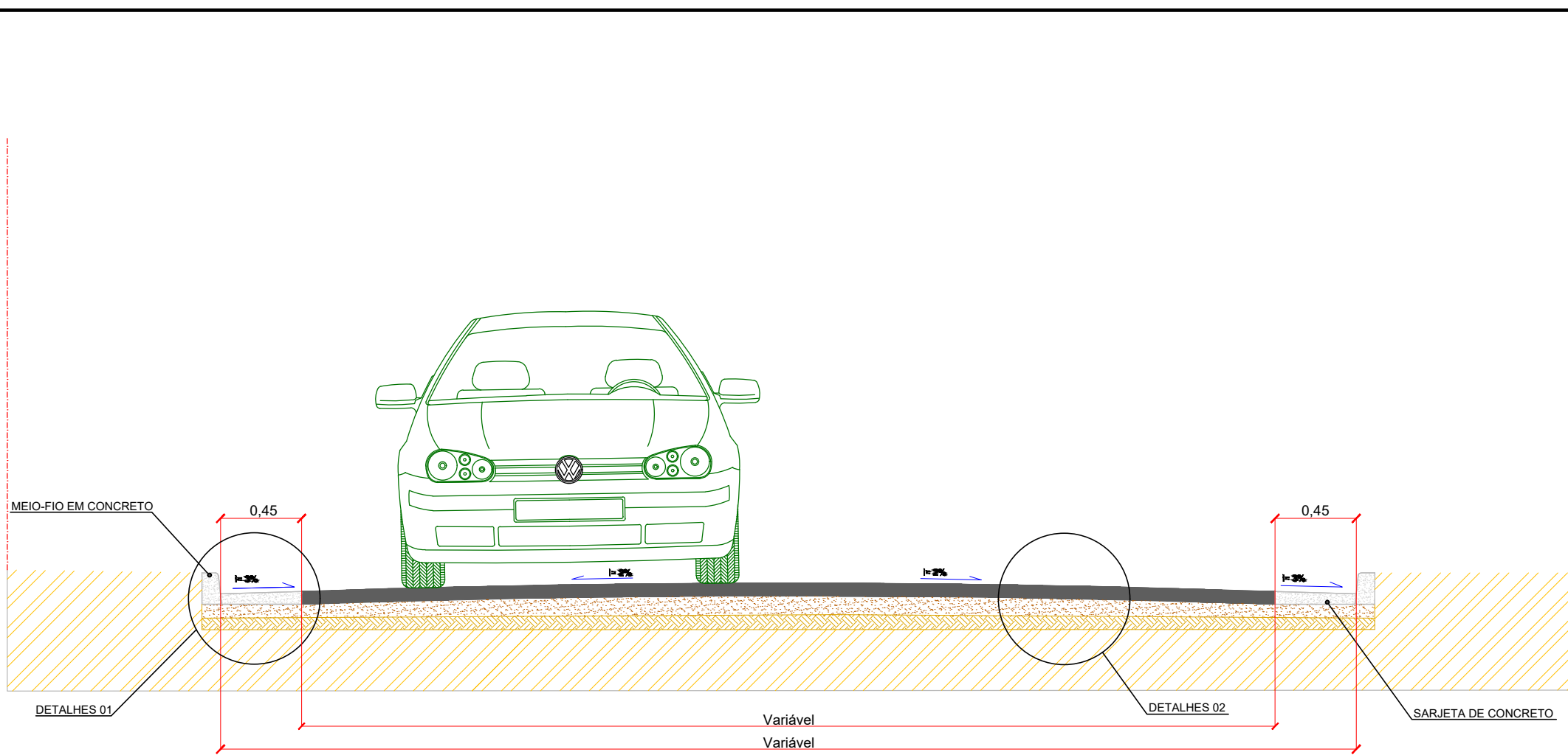
Corte Transversal - Pista de Rolamento - Implantação Asfáltica Escala: sem escala Cota: m
