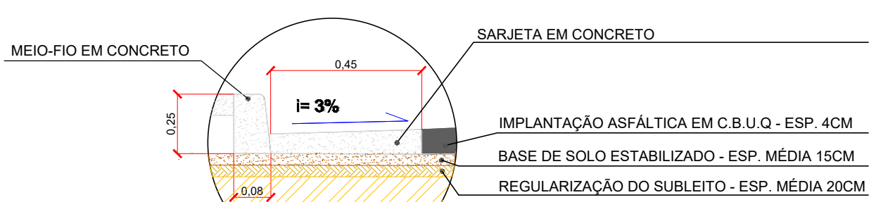
Detalhe 01 Sem Escala Cota: m
