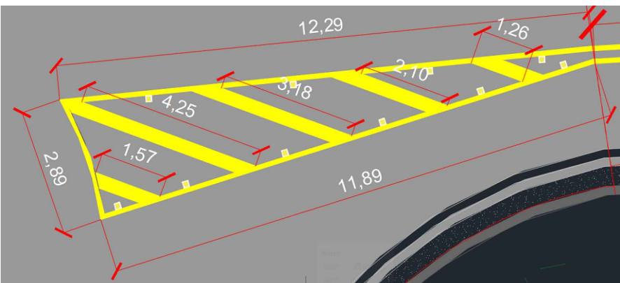
Detalhamento da zebra de preenchimento da área de pavimento não utilizável Cotas: m Linhas de 0,30m = 12,36m x 0,30m = 3,708m² Linhas de 0,10m = 27,07m Tachas refletivas: 10 unidades
