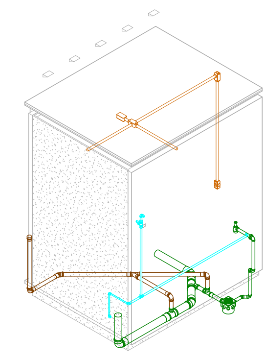
8 ISO - ÁREA MOLHADA 06 ESCALA
