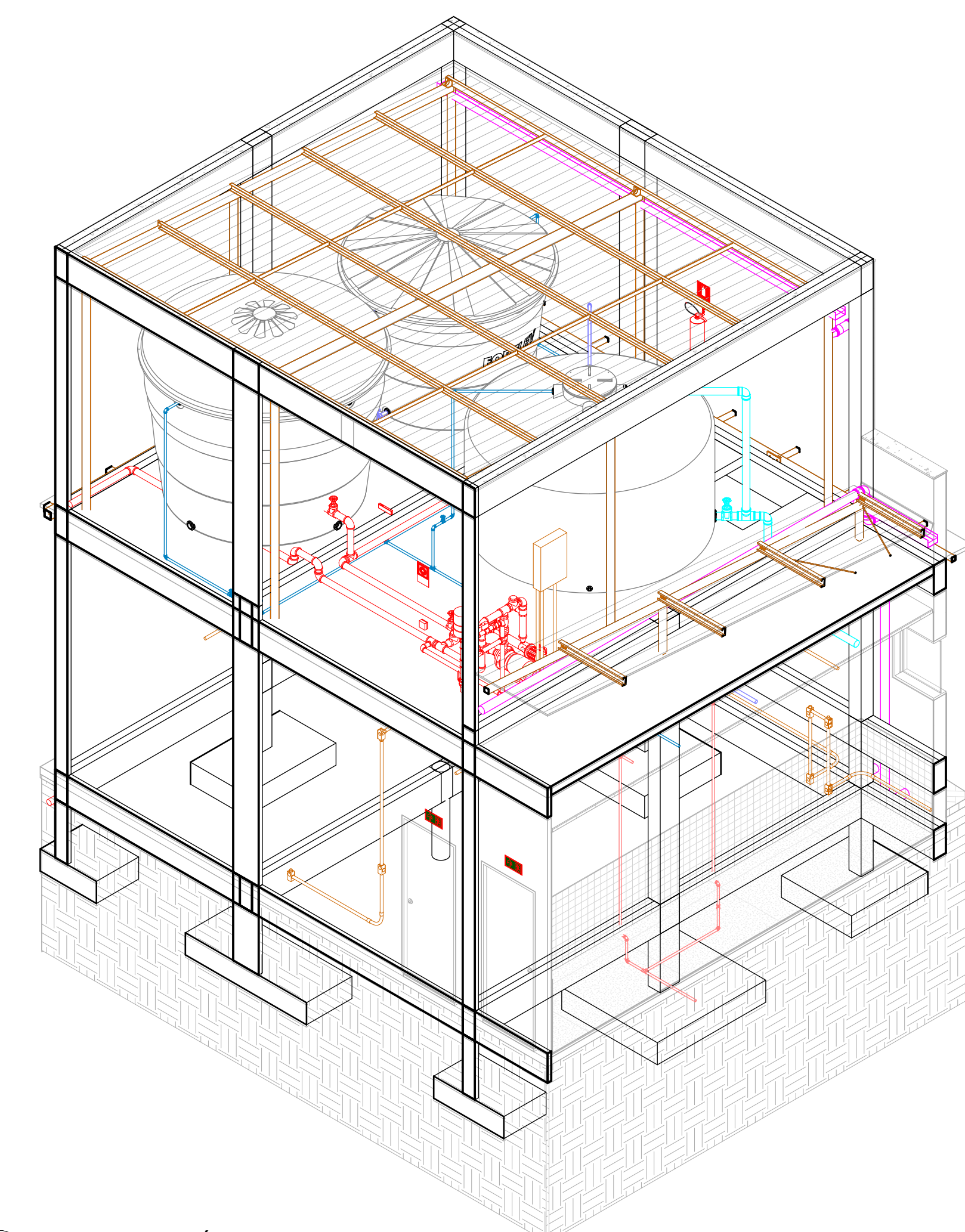
2 ISO - CAIXA D'ÁGUA ESCALA
