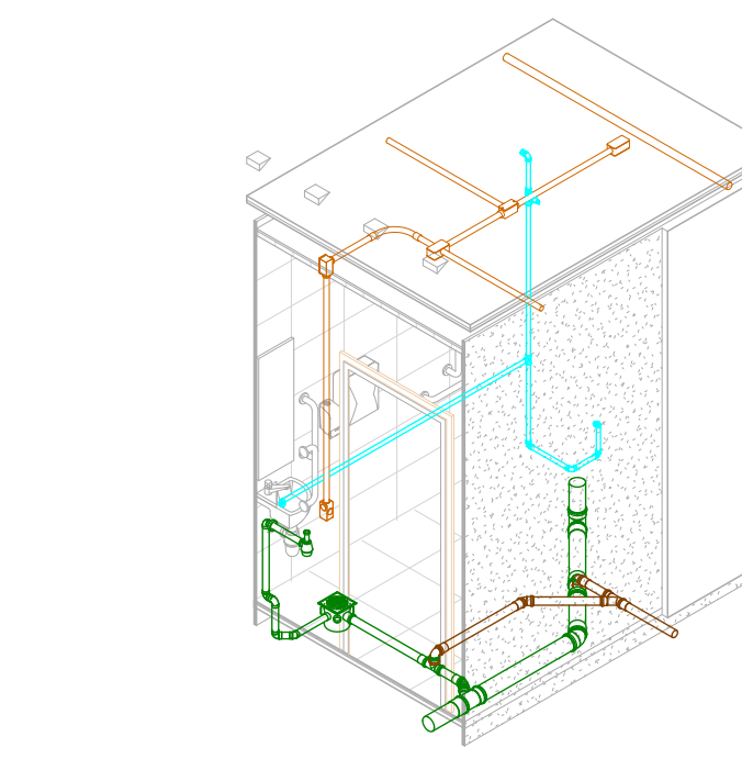
9 ISO - ÁREA MOLHADA 07 ESCALA
