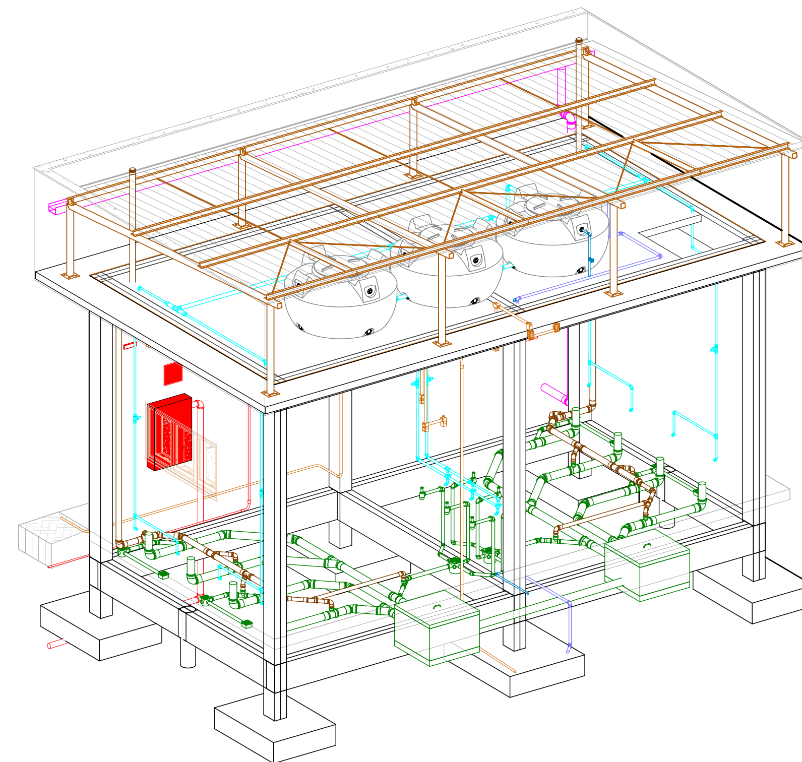
2 ISO - ÁREA MOLHADA 08 COMPLETA ESCALA
