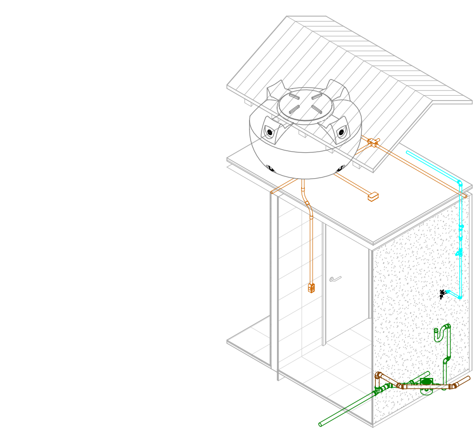
2 ISO - ÁREA MOLHADA 01 ESCALA
