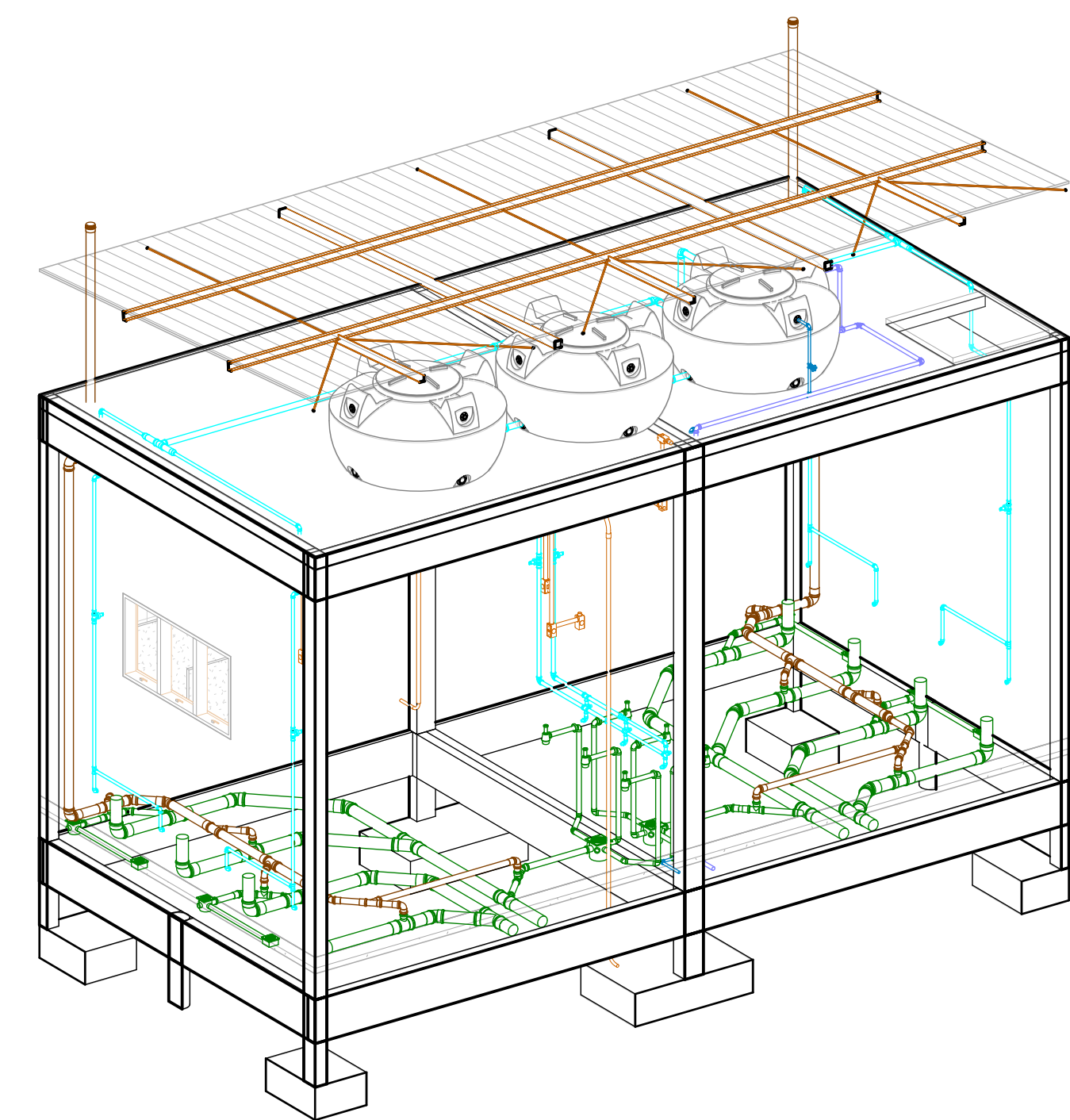
3 ISO - ÁREA MOLHADA 08 ESCALA
