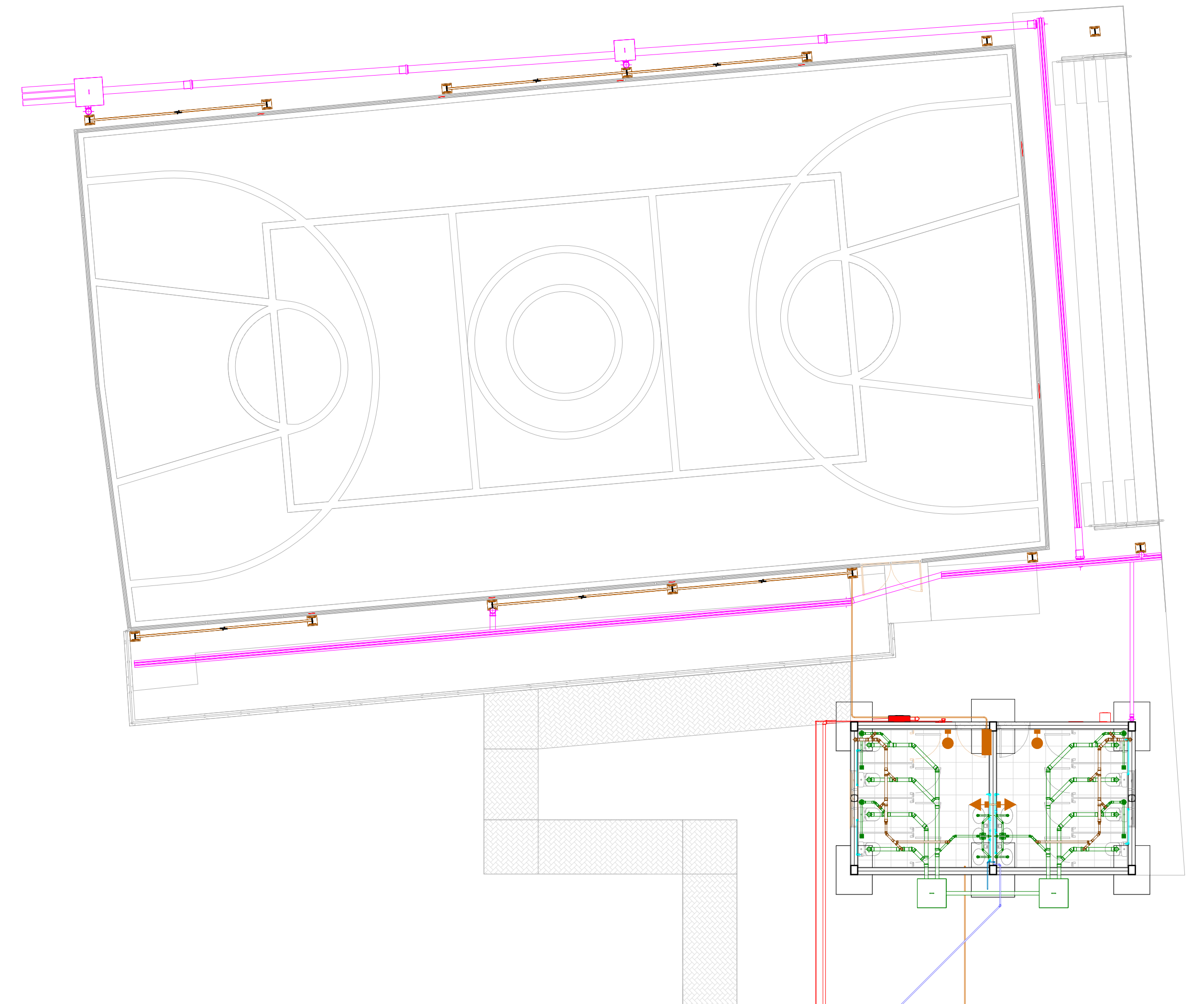
2 004 - CTZ - FUNDAÇÃO QUADRA ESCALA 1:100
