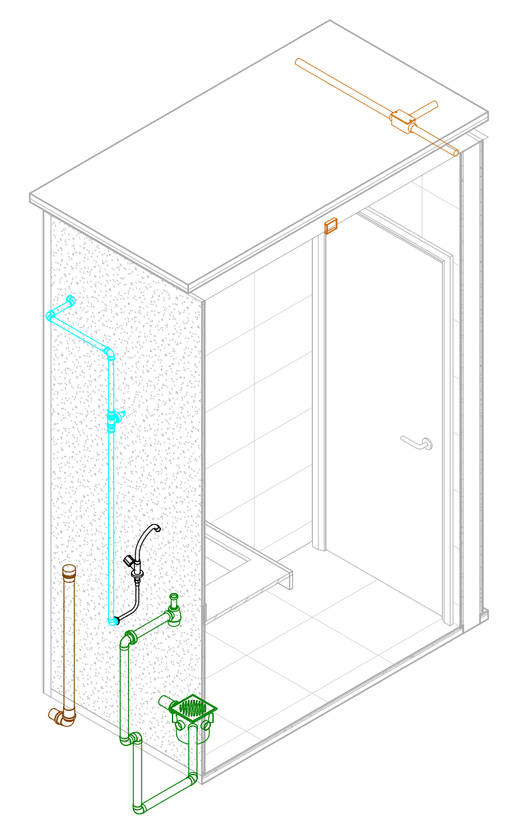
3 ISO - ÁREA MOLHADA 02 ESCALA
