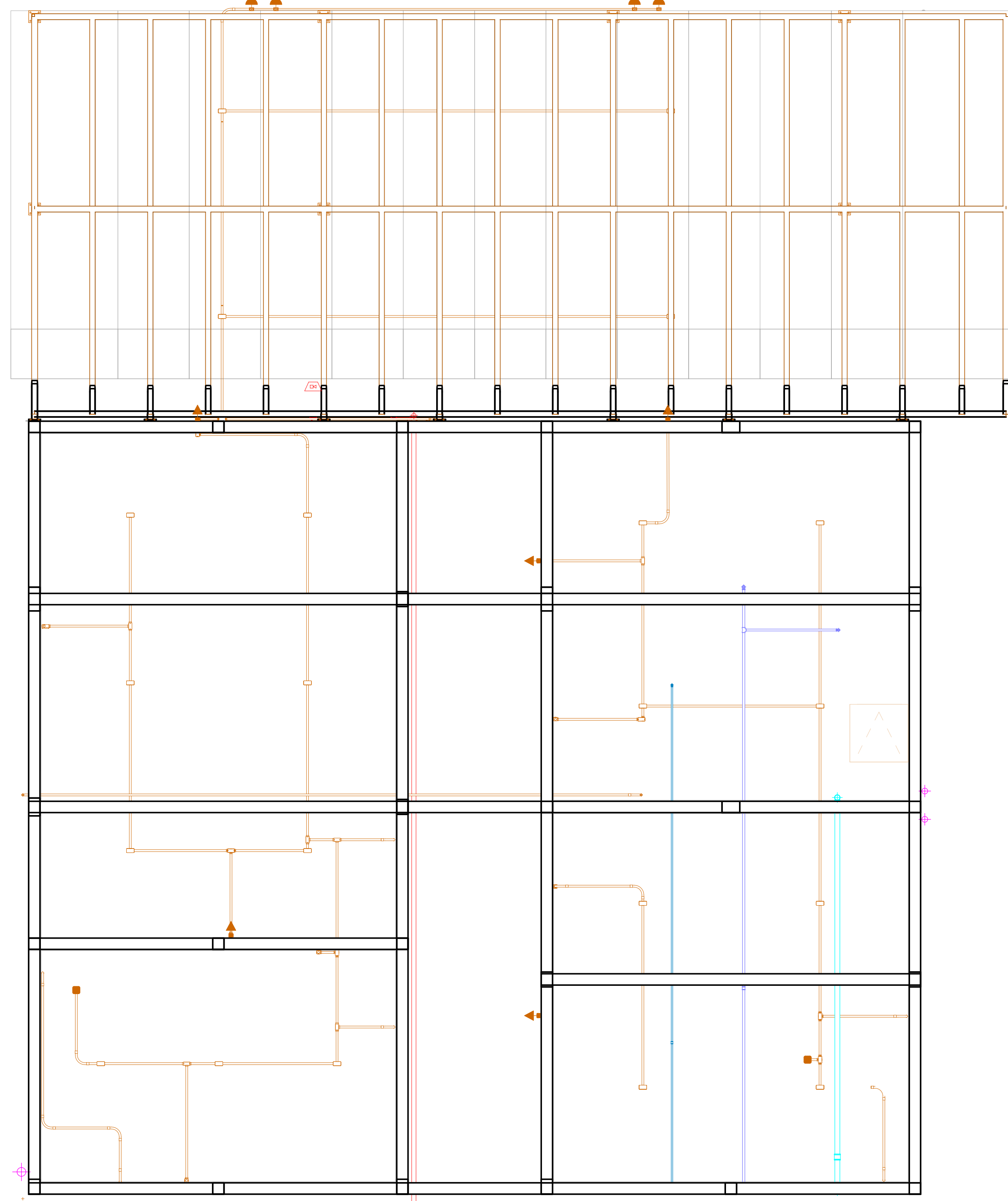
4 000 - CTZ - ENTREFORÇO TÉRREO ESCALA 1:50
