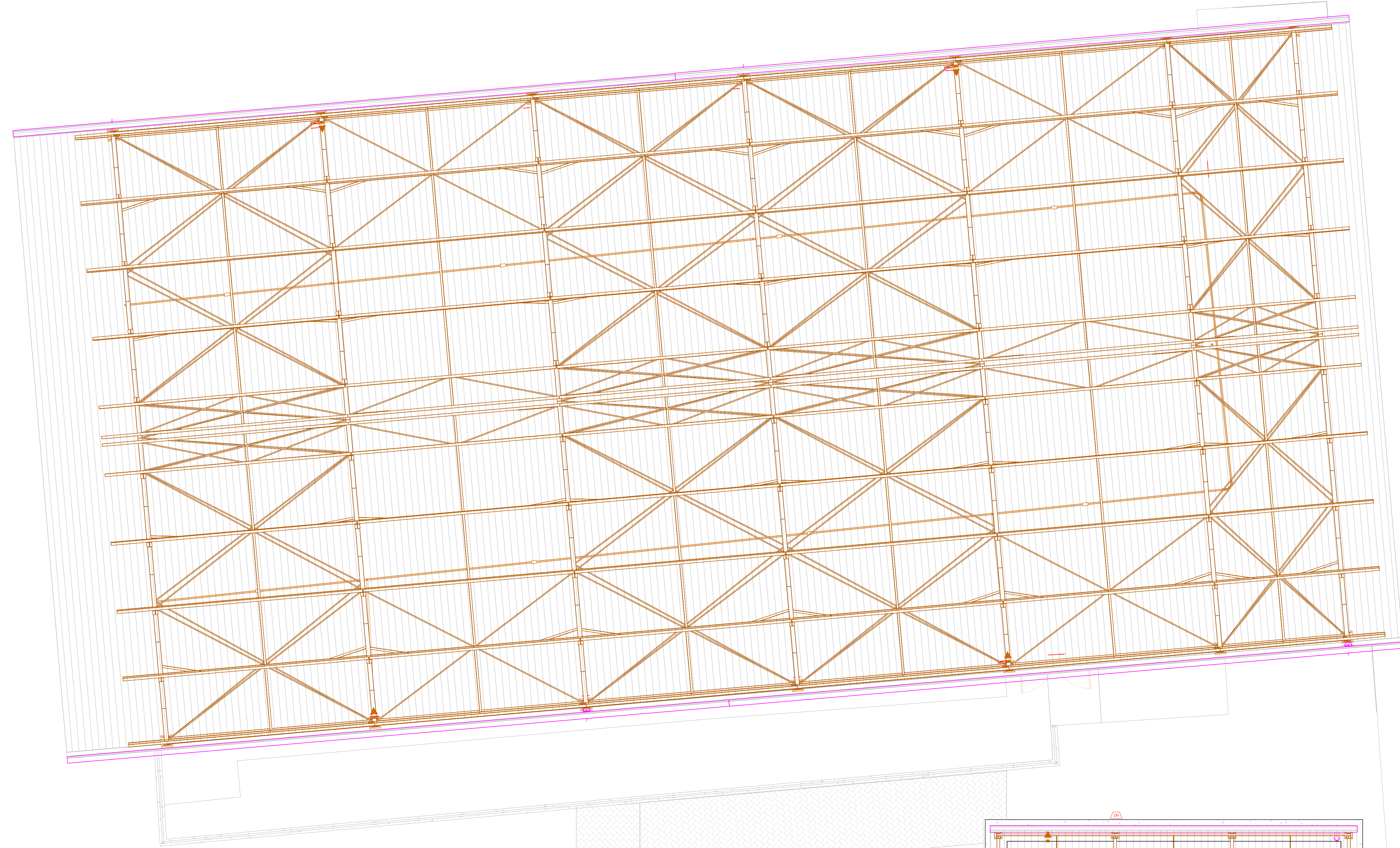
003 - CTZ - ENTREFORRO QUADRA ESCALA 1:50
