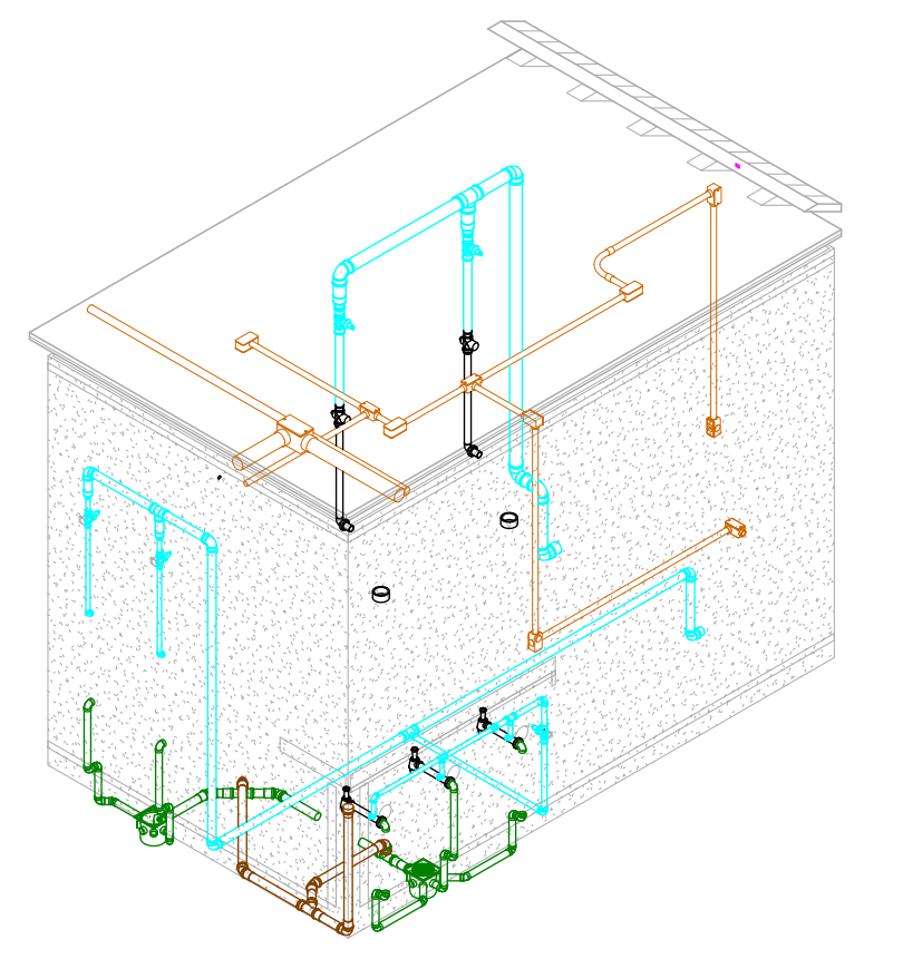
6 ISO - ÁREA MOLHADA 04 ESCALA
