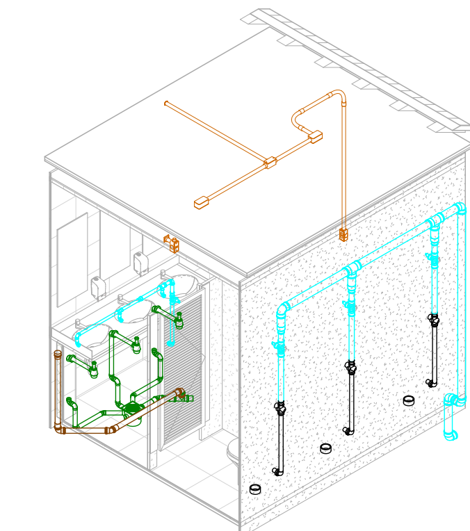
7 ISO - ÁREA MOLHADA 05 ESCALA
