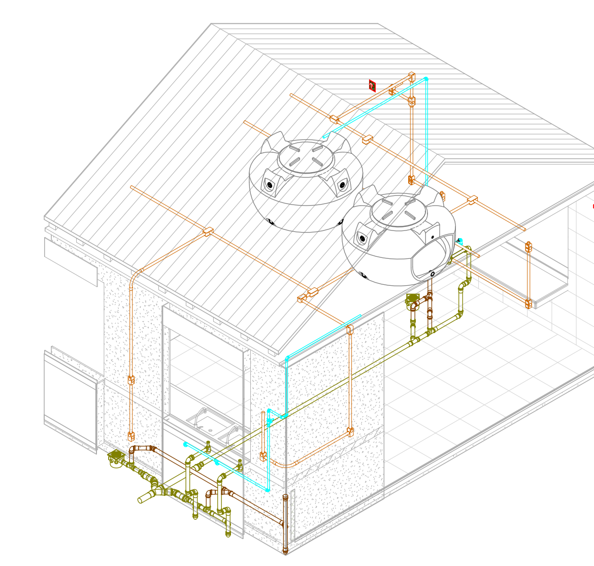
5 ISO - ÁREA MOLHADA 03 ESCALA
