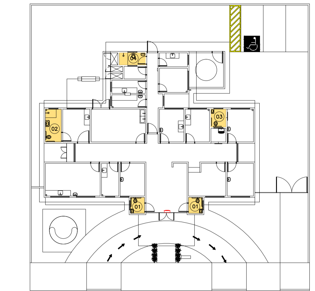
Planta Esquemática de Localização de Detalhes UBS 1 Nível: 0,00m Sem Escala Detalhe Desnível ESCALA 1:5
